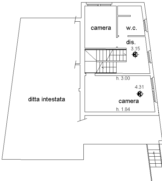
Pianta piano primo h. 2.76
