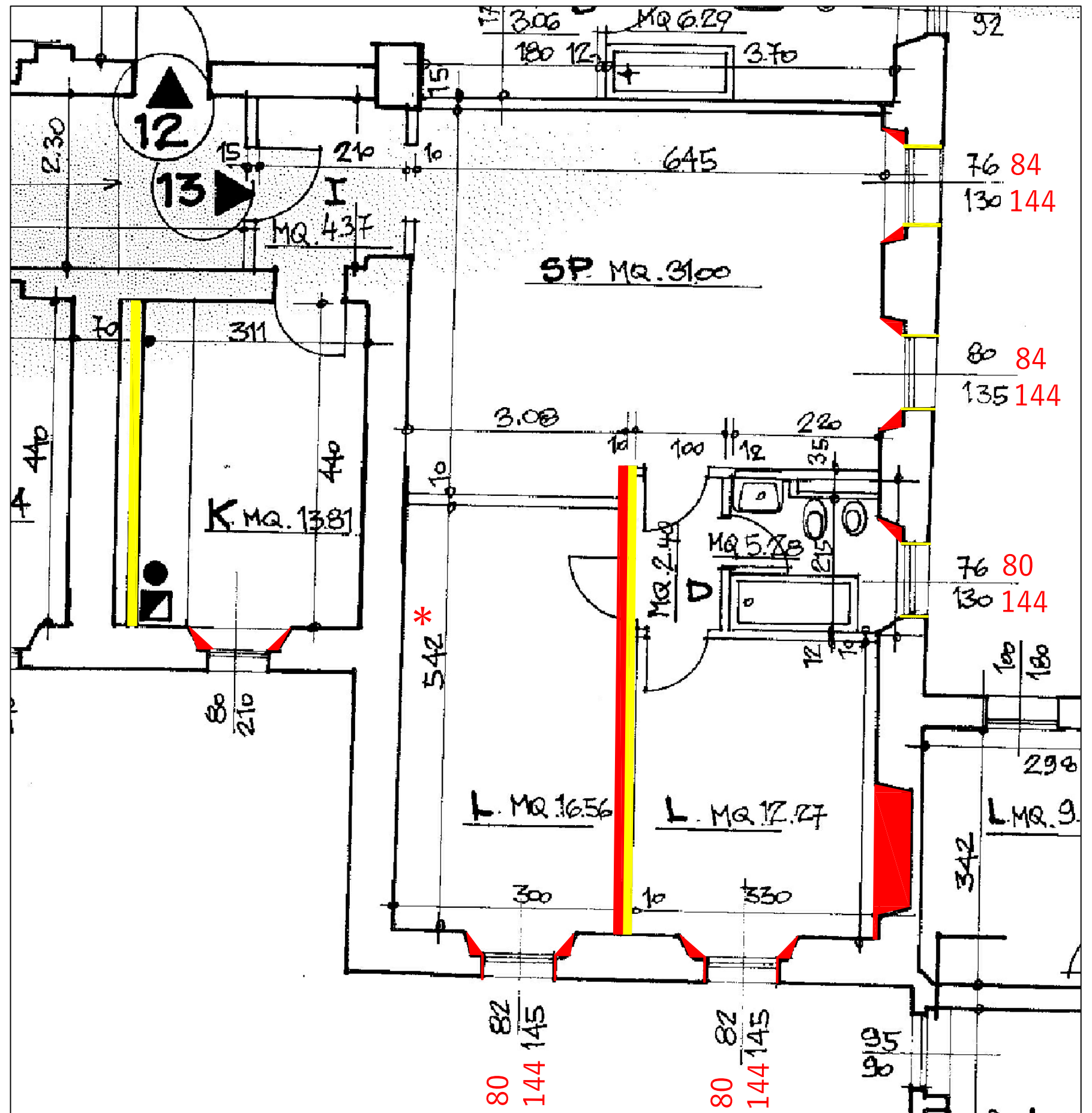
Appartamento - Piano 3
